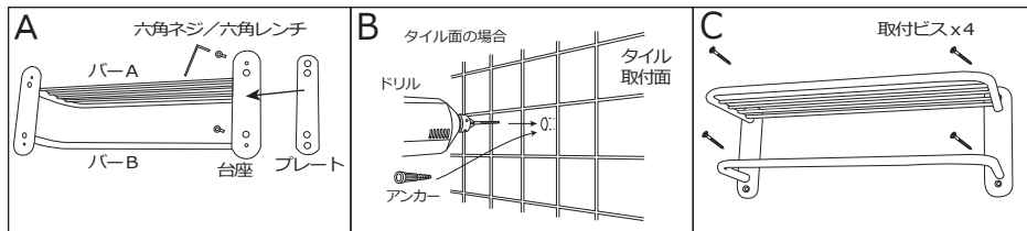
A 台座にプレートをはめて、バーAとバーBを裏から六角レンチにて締め付けて、本体を組み立てます。 B タイル面に取付ける場合は、ビスを取付ける位置にドリルで穴を開け、付属の樹脂製アンカーを挿入します。 C 付属の取付ビスにて、壁面に固定して下さい。タイル面の場合は先に位置決めしたアンカーへ取付けてください。
