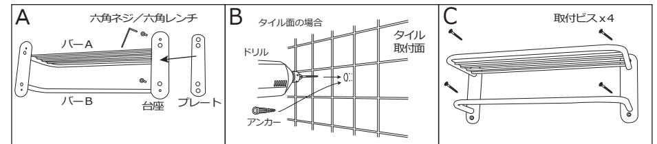
A 台座にプレートをはめて、バーAとバーBを裏から六角ネジと六角レンチにて締め付けて、本体を組み立てます。 B タイル面に取付ける場合は、ビスを取付ける位置にドリルで穴を開け、付属の樹脂製アンカーを挿入します。 C 付属の取付ビスにて、壁面に固定して下さい。タイル面の場合は先に位置決めしたアンカーへ取付けてください。
